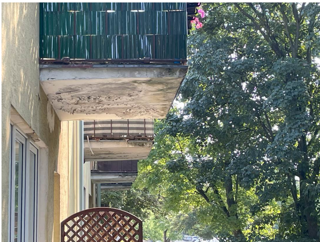
Fot. 4. Widok uszkodzeń płyty balkonowej.
